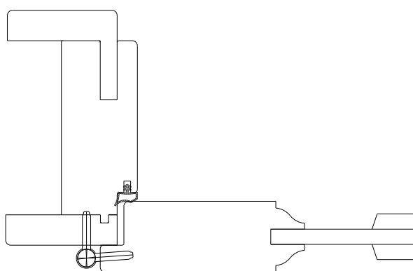
drzwi wewnętrzne przylgowe
