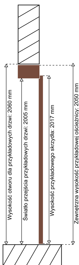
wymiarowanie wysokości drzwi
