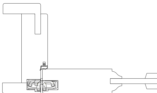
drzwi wewnętrzne bezprzylgowe
