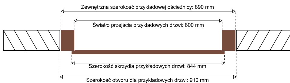
wymiarowanie szerokości drzwi
